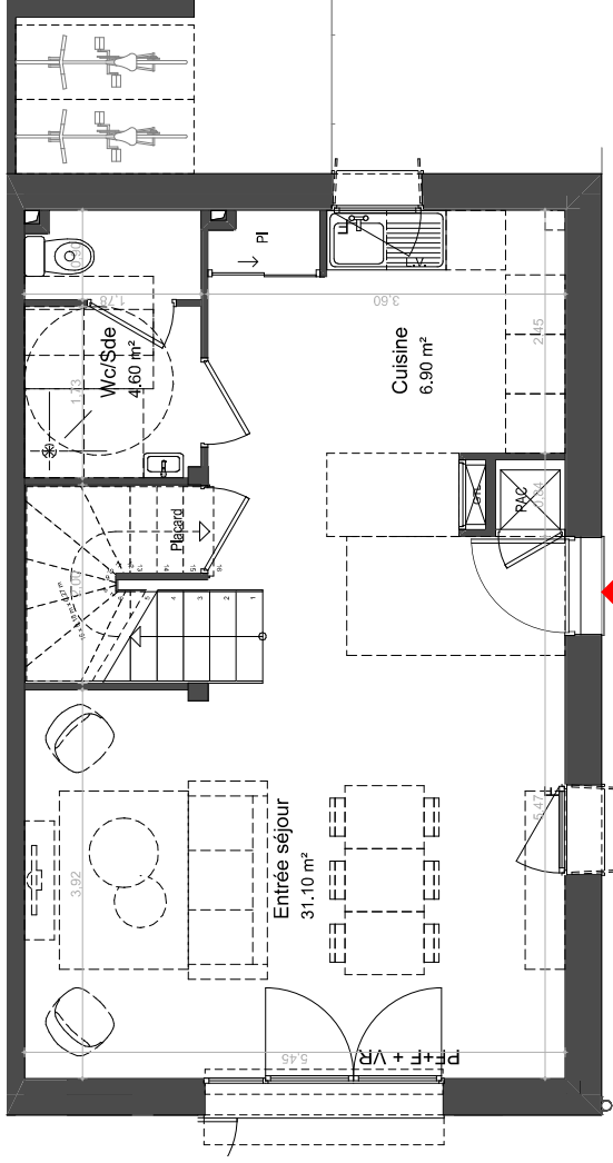
Plan de ROC
