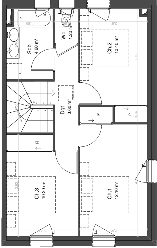
Plan de R+1
